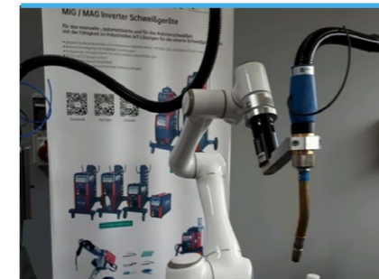
Megmeet welder
